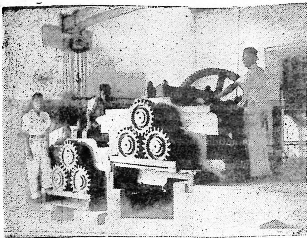
Este engenho é notável pela sua eficiência. Fora do comum é serrado por 6 moendas numa engrenagem dupla, oferecendo um aproveitamento máximo do caldo da cana (vide página anterior).
